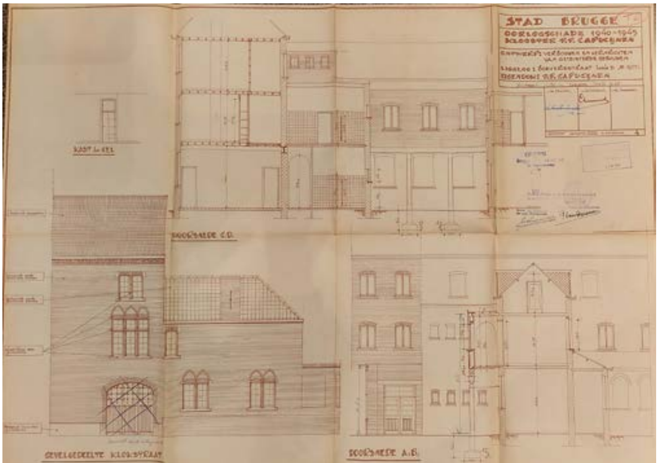
25. Plan ontwerp gevel Kloosterstraat en doorsnedes voor herstel oorlogsschade, architect Emiel Allewaerts, feb. 1947 (Stadsarchief Brugge, bouw-aanvraag 1947/361)
