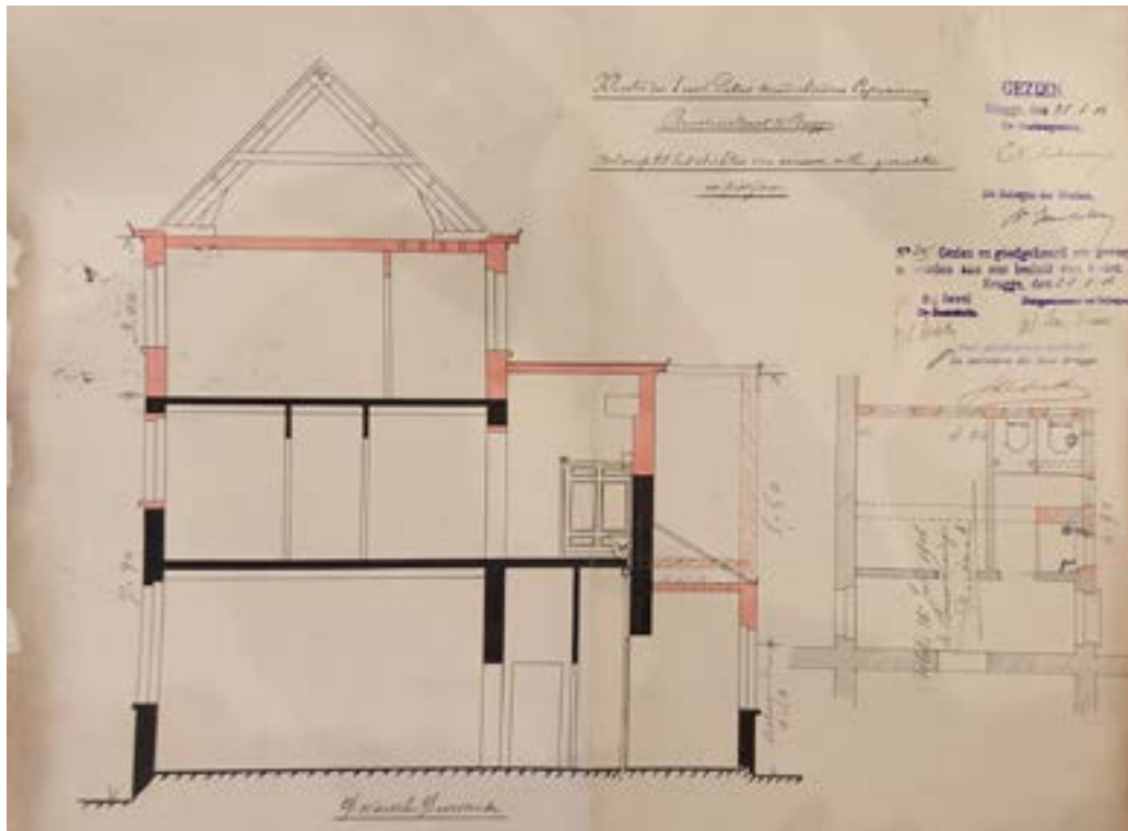
14. Plan bij bouwaanvraag 1906/245 voor 'stichten van nieuwe cellen, gemakken en pissijnen - dwarsche doorsnede", architect J. Goethals (Aalst) (Stadsarchief Brugge)
