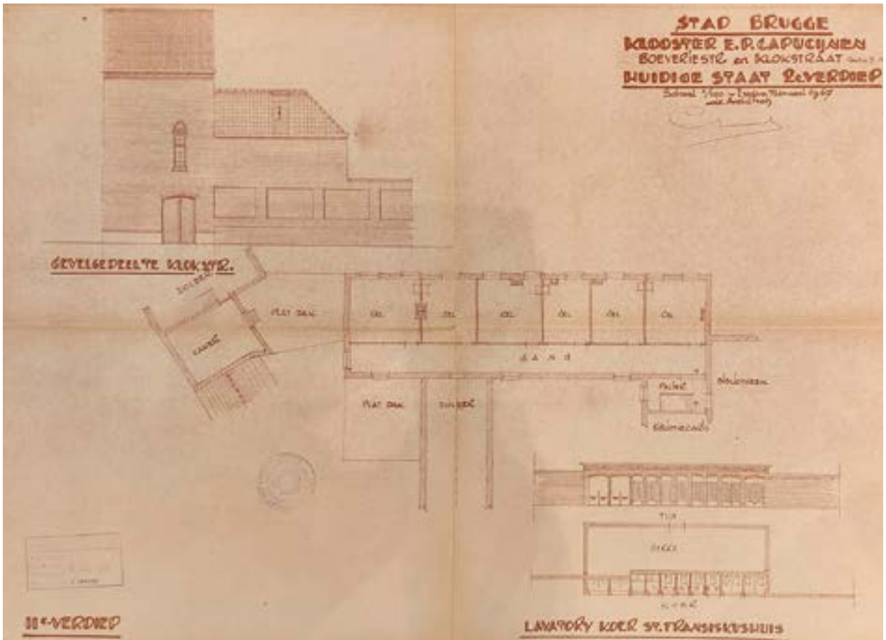
23. Plan bestaande toestand 2de verdiep voor herstel oorlogsschade, architect Emiel Allewaerts, feb. 1947 (Stadsarchief Brugge, bouw-aanvraag 1947/361)
