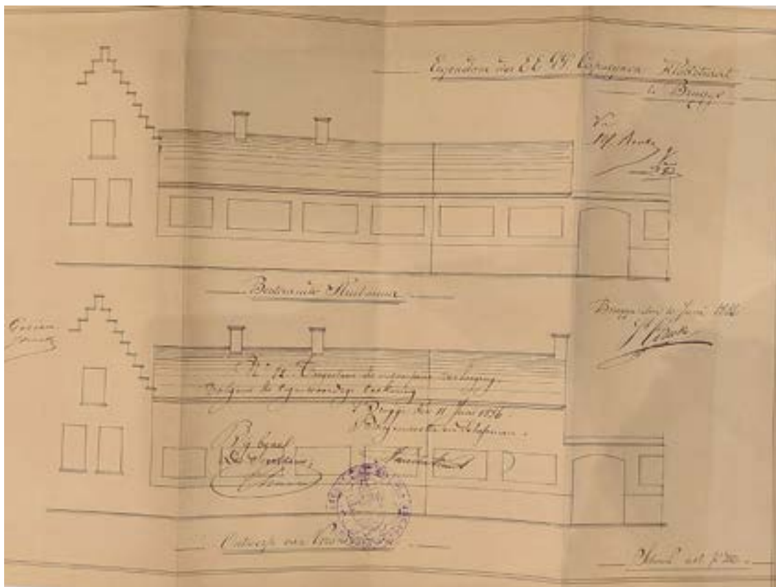
05. Plan bij bouwaanvraag 1886/72 voor de veranderingen aan de Klokstraat (bouw vleugel en verhoging afsluitingsmuur), architect Jh. Coucke, 10 juni 1886 (Stadsarchief Brugge)
