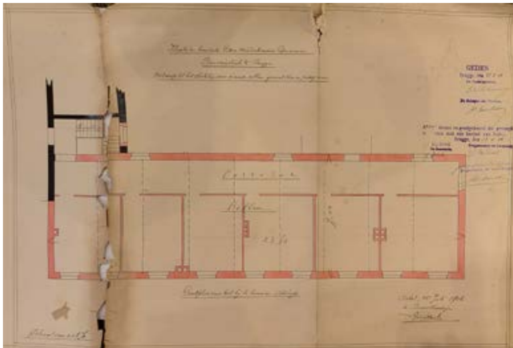
15. Plan bij bouwaanvraag 1906/245 voor 'stichten van nieuwe cellen, gemakken en pissijnen - grondplan van het bij te bouwen verdiep , architect Goethals (Stadsarchief Brugge)
