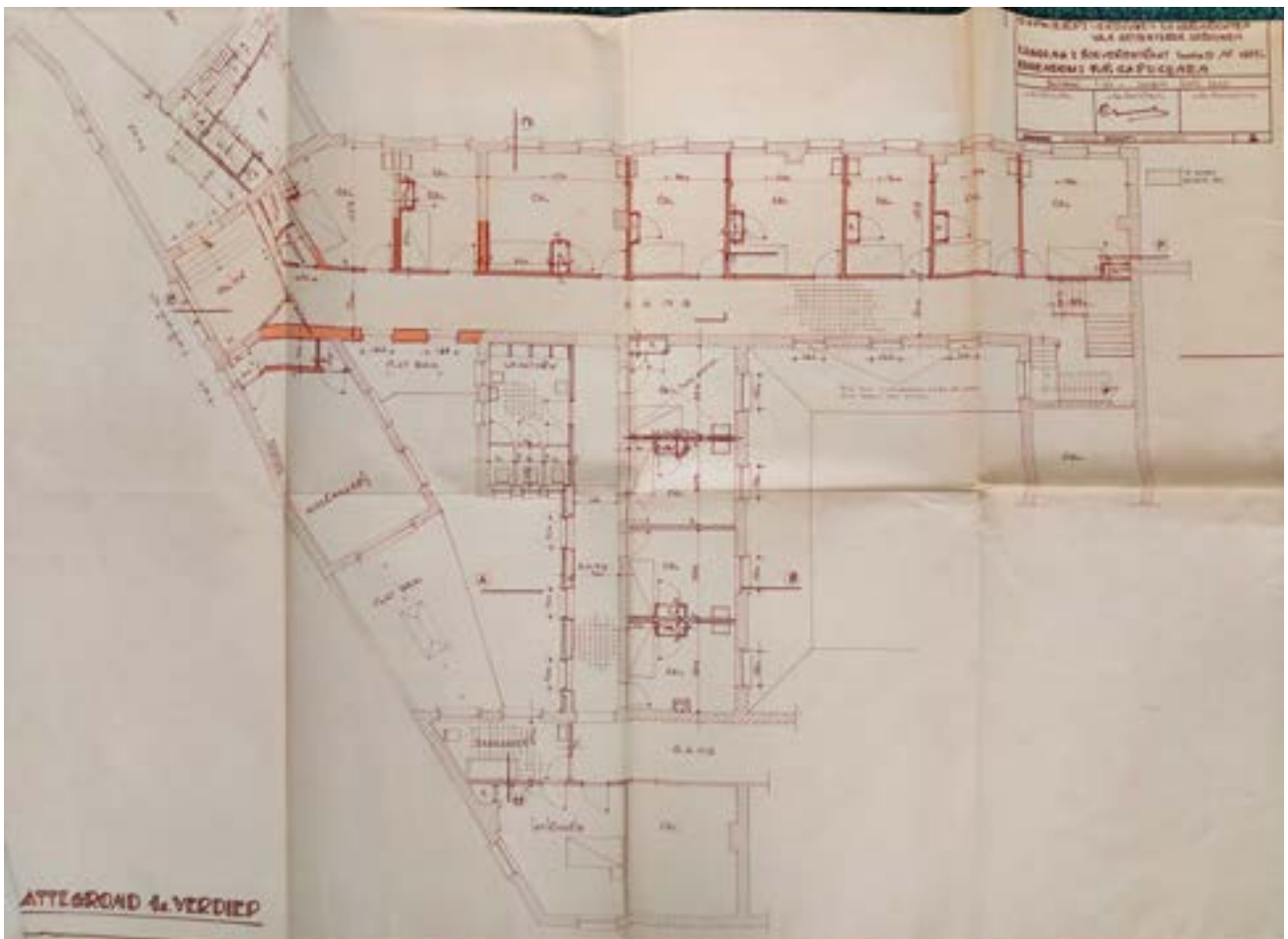
22. Plan ontwerp 1ste verdiep voor herstel oorlogsschade, architect Emiel Allewaerts, feb. 1947 (Stadsarchief Brugge, bouwaanvraag 1947/361)
