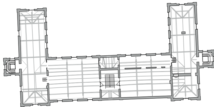
NIVEAU 0 KOETSHUIS
