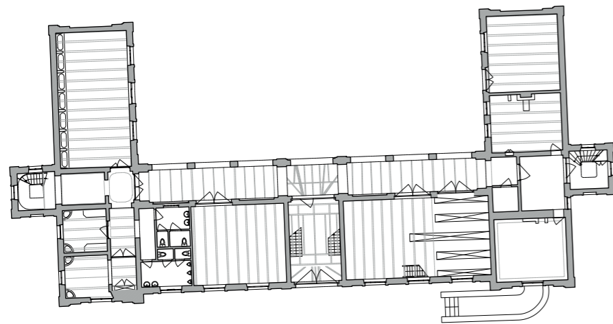
NIVEAU 0 KOETSHUIS
