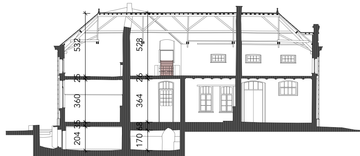
Koetshuis doorsnede BB'
