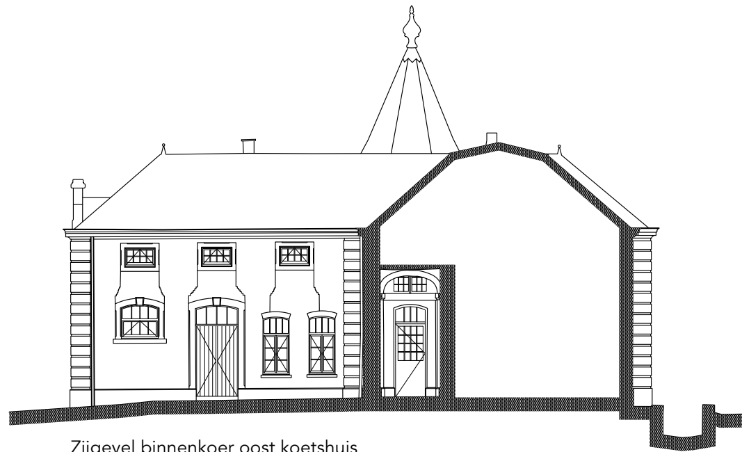
Zijgevel binnenkoer oost koetshuis
