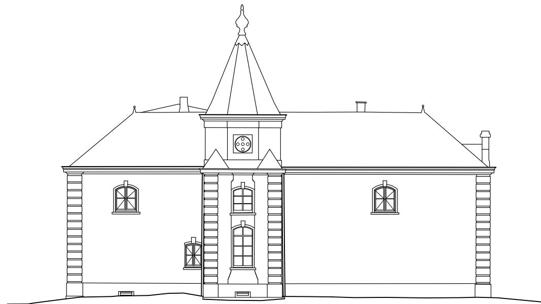
Zijgevel rechts koetshuis
